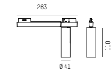
ROGGA SHORT DC Volare 6,5 - 12W 300-1220lm
